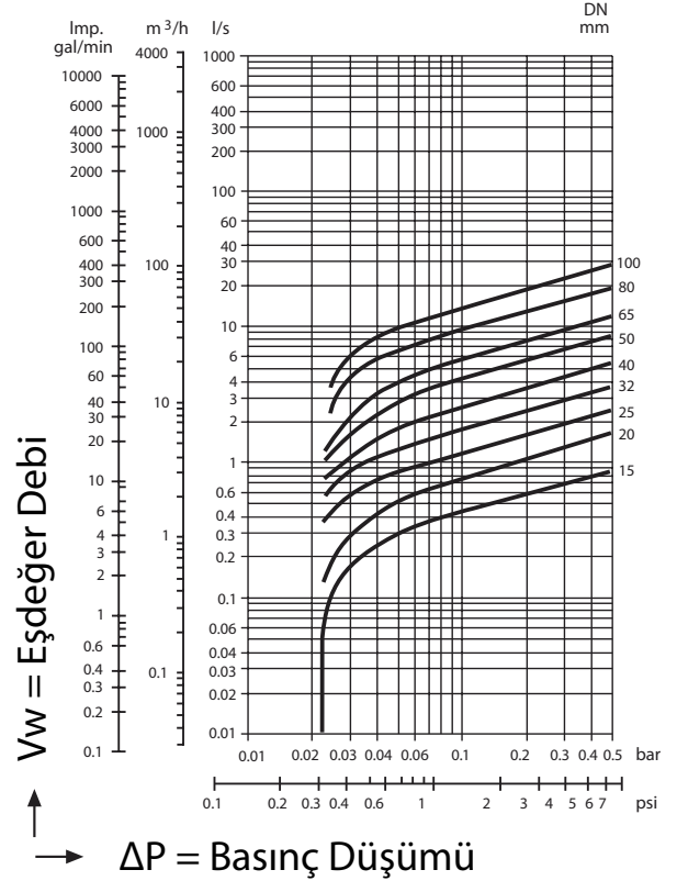
Basınç Düşümü Grafiği
